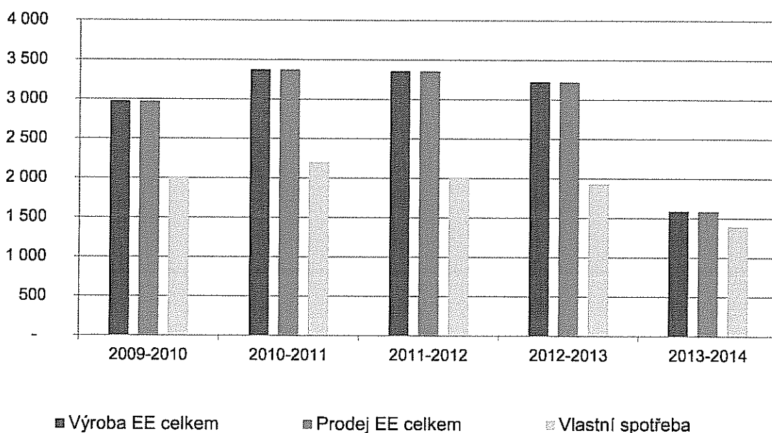
Výroba a prodej elektrické energie 2009 – 2014 (v MWh)
